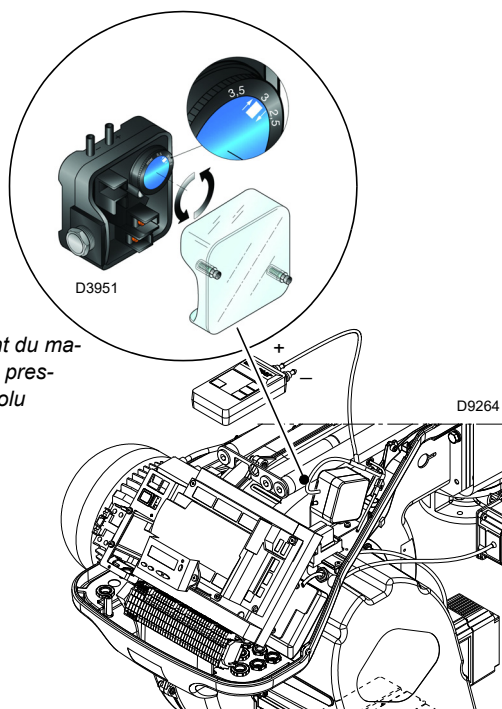
Raccordement du manomètre avec pressostat en différentiel
