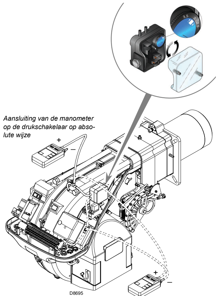
Aansluiting van de manometer op de drukschakelaar op differentiële wijze
