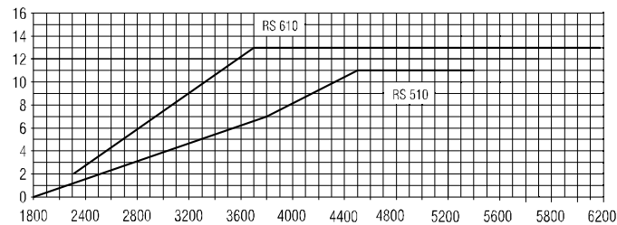
Максимальная мощность горелки (кВт) Рис. 19
