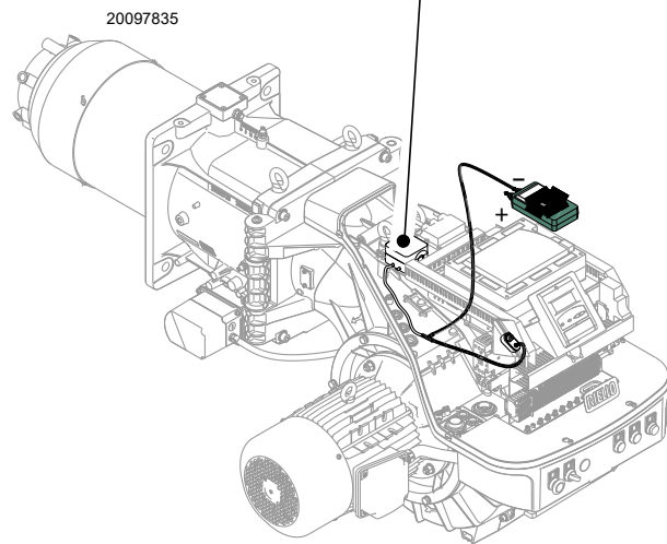
Anschluss des Druckmessers mit Absolut-Druckwächter
