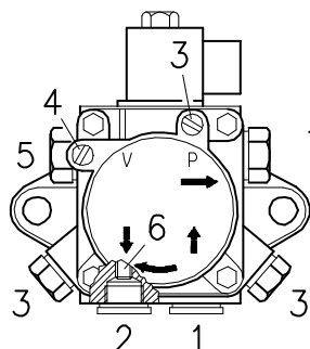
RL 70 PUMPE SUNTEC AL 95 C
