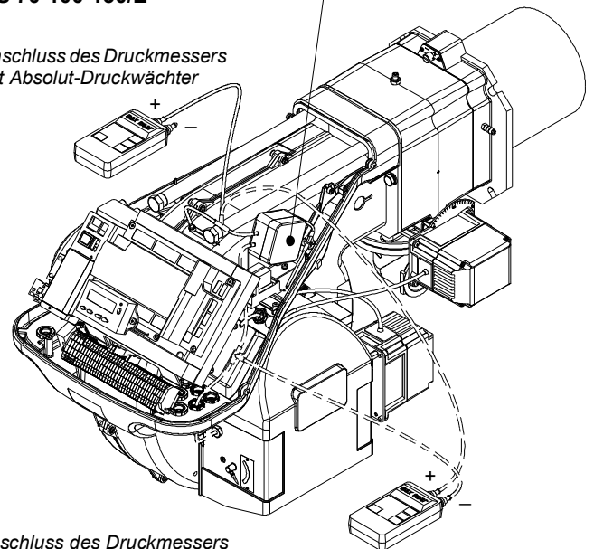
Anschluss des Druckmessers mit Differential-Druckwächter
