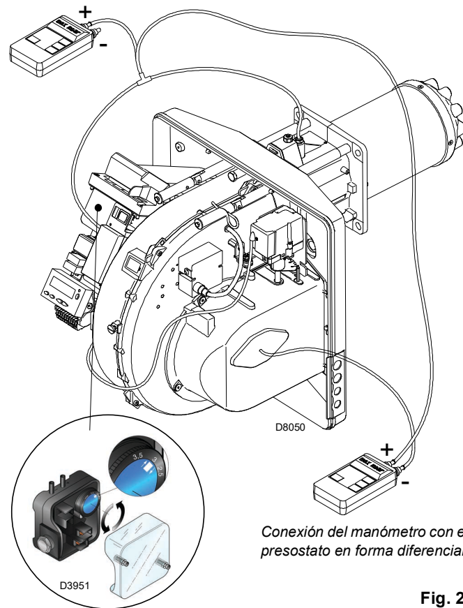
Conexión del manómetro con el presostato en forma absoluta
