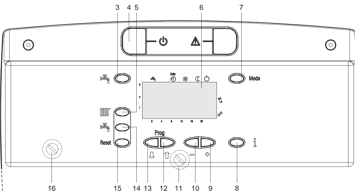
ЩИТ УПРАВЛЕНИЯ В ОТКРЫТОМ СОСТОЯНИИ
