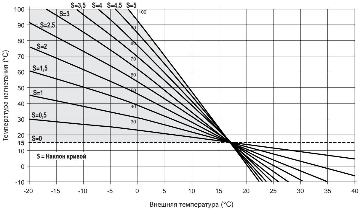
Температурные кривые для уставки температуры в помещении 15°C
