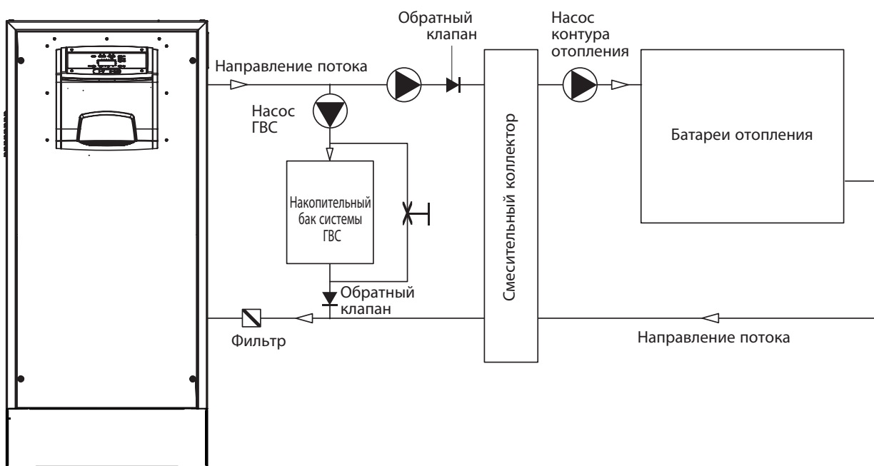
Котел с контуром ГВС (тепло котла > горячая вода для ГВС) и 1 группой батарей отопления
