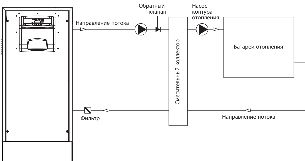
Котел с группой радиаторов отопления
