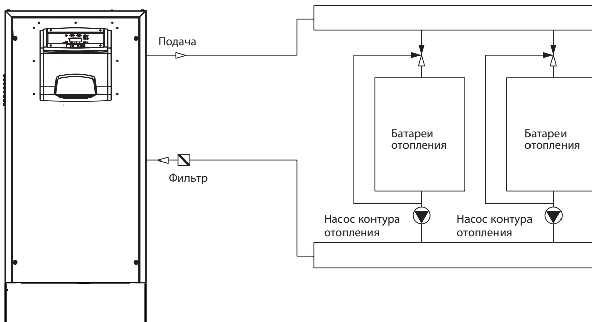
Котел с несколькими группами радиаторов отопления
