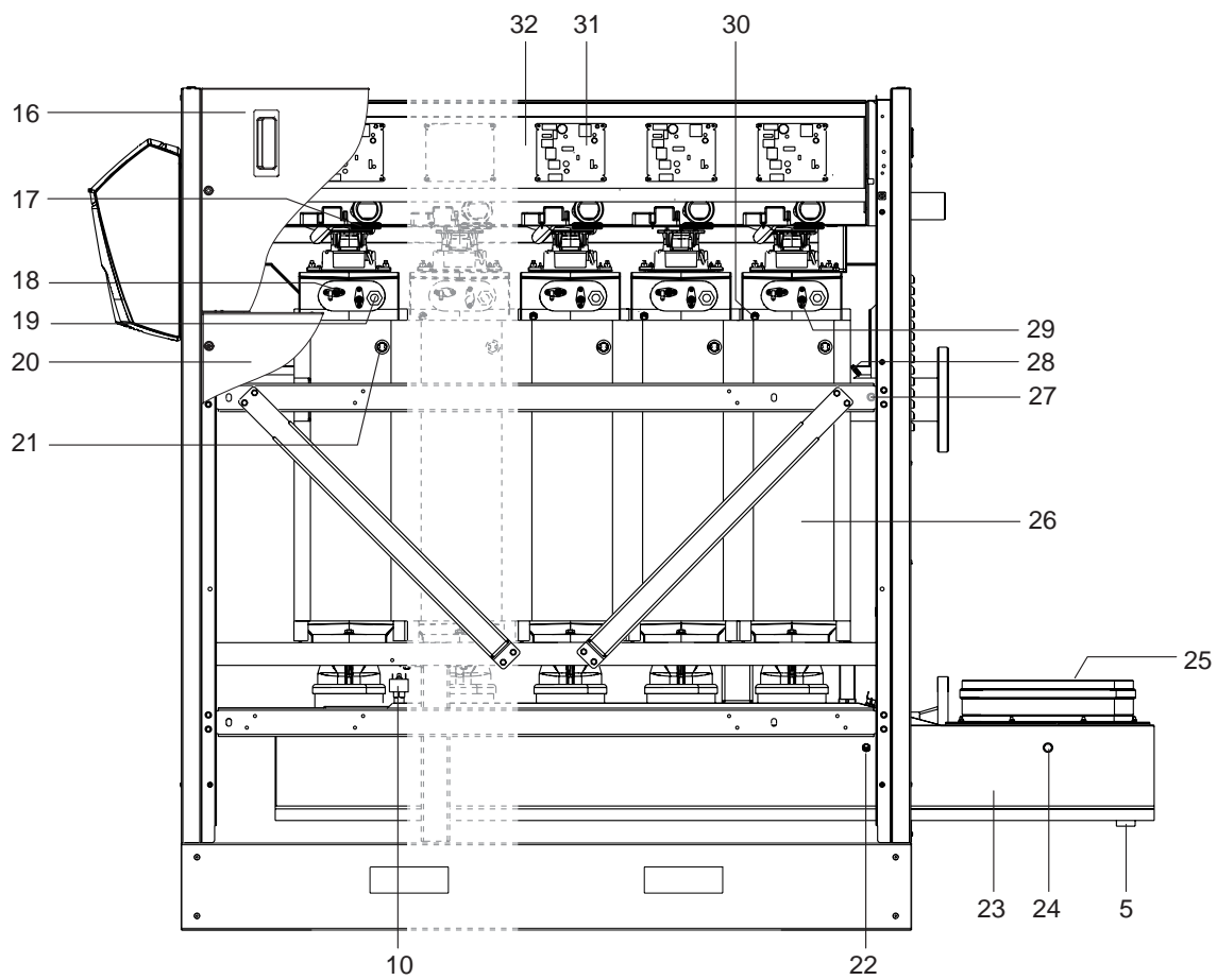
Вид СПРАВА
