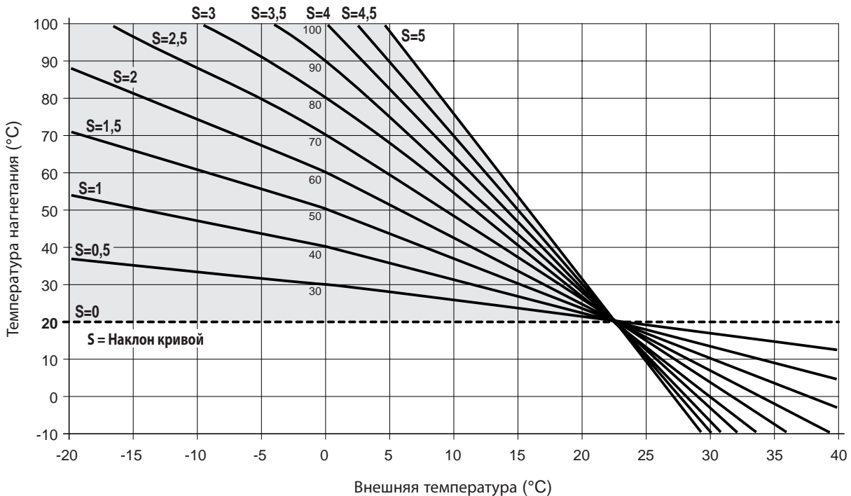
Температурные кривые для уставки температуры в помещении 20°C
