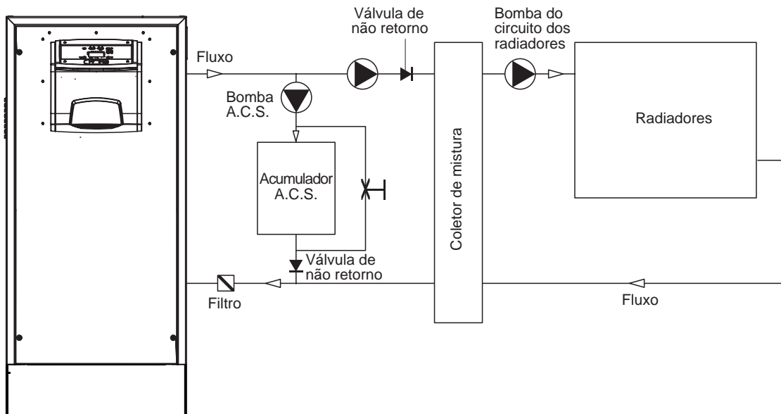
Circuito da caldeira com bomba A.C.S. (produção caldeira > produção A.C.S.) e 1 grupo de radiadores
