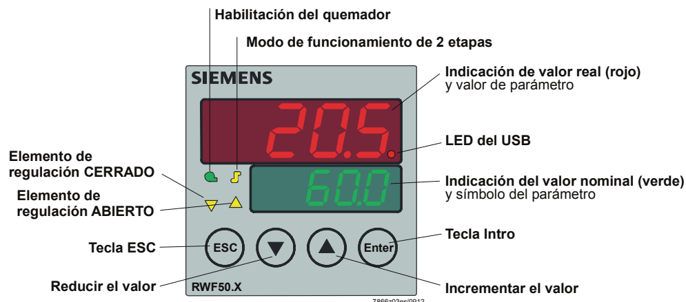
Figura 16: Significado de las indicaciones y de las teclas
