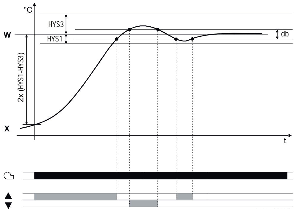
Figura 14: Secuencia de control del arranque en frío de una instalación
