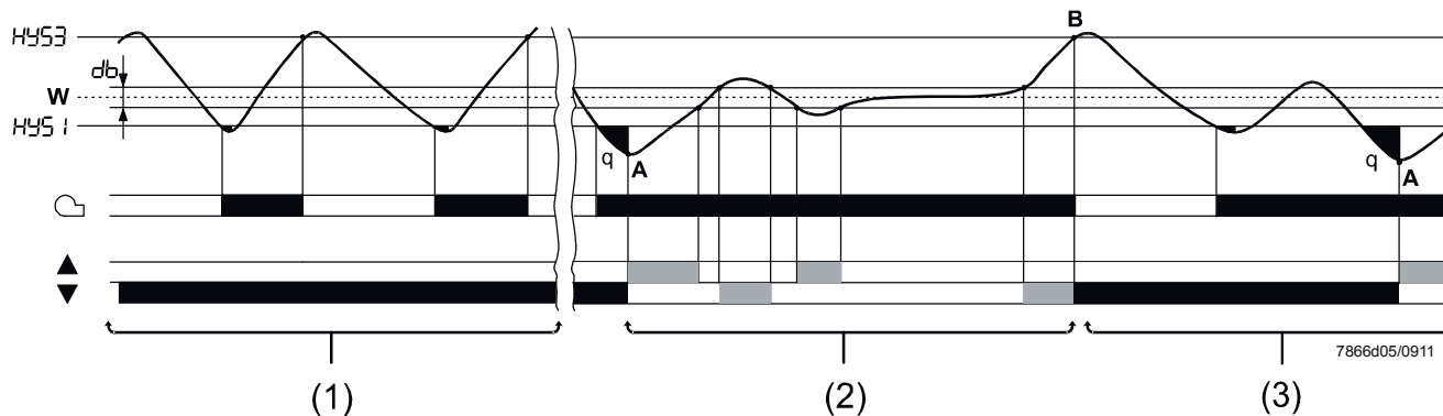
Afbeelding 8: Programmaverloop brander modulerend 3-puntsuitgang
