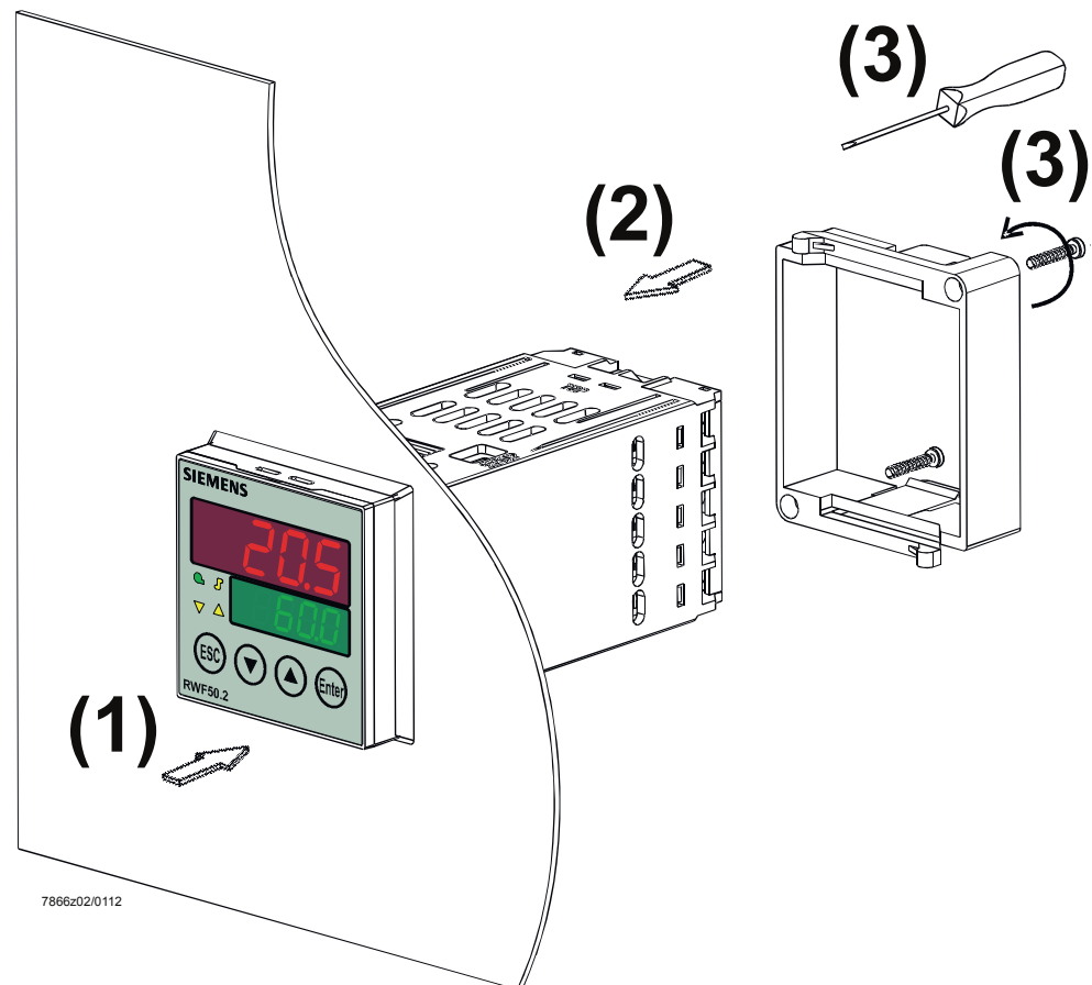
Afbeelding 3: Inbouw in schakepaneeluitsparing
