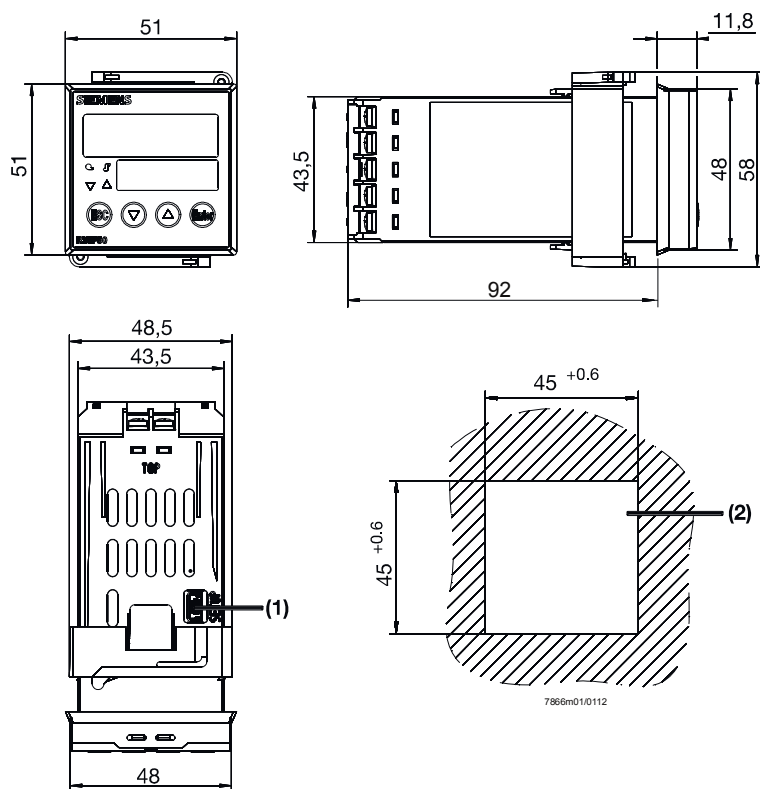
Afbeelding 2: Afmetingen RWF50
