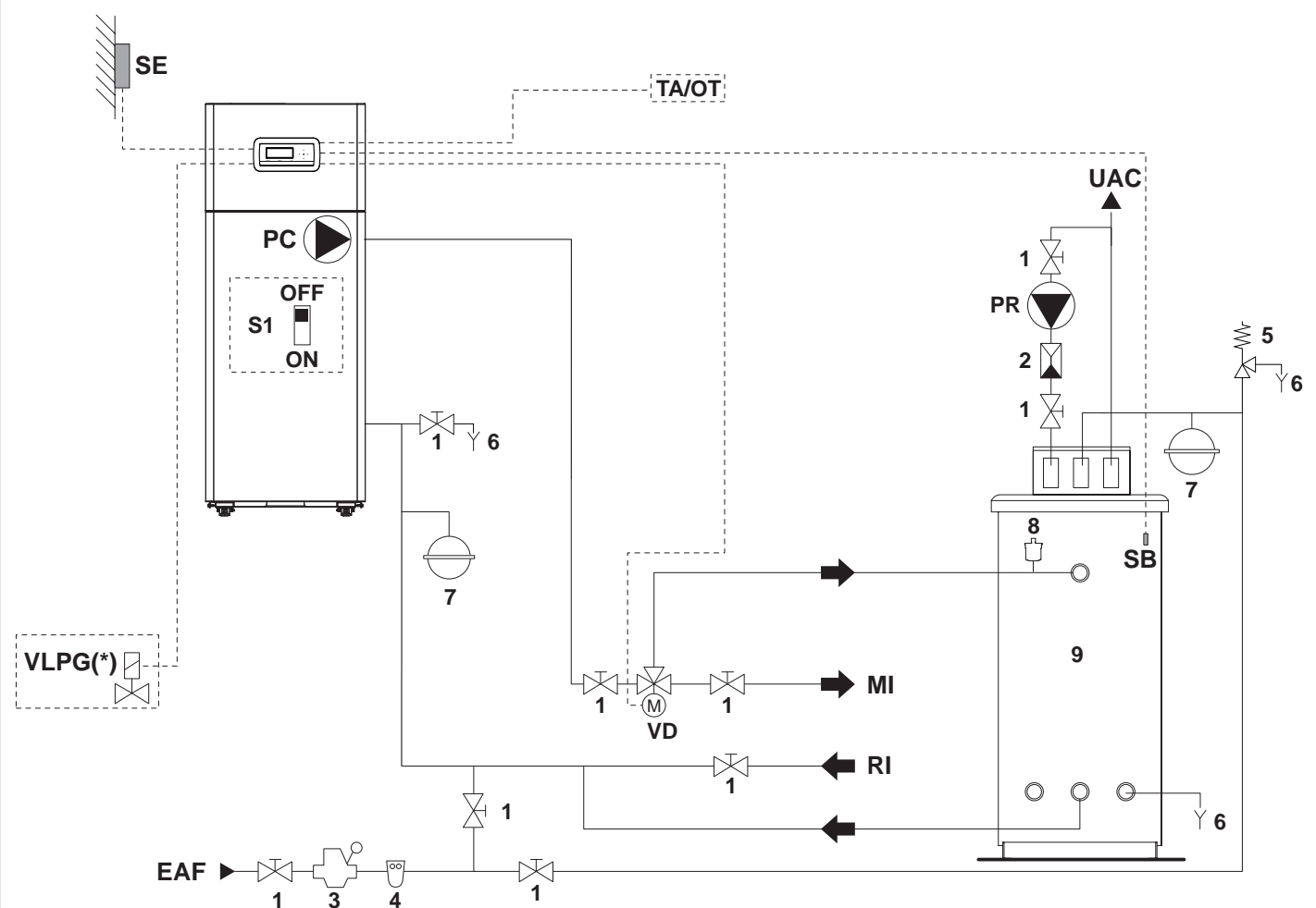
Schéma 2 : circuit avec module thermique connecté directement à l'installation de chauffage et production d'ECS avec chauffe-eau et vanne déviatrice
