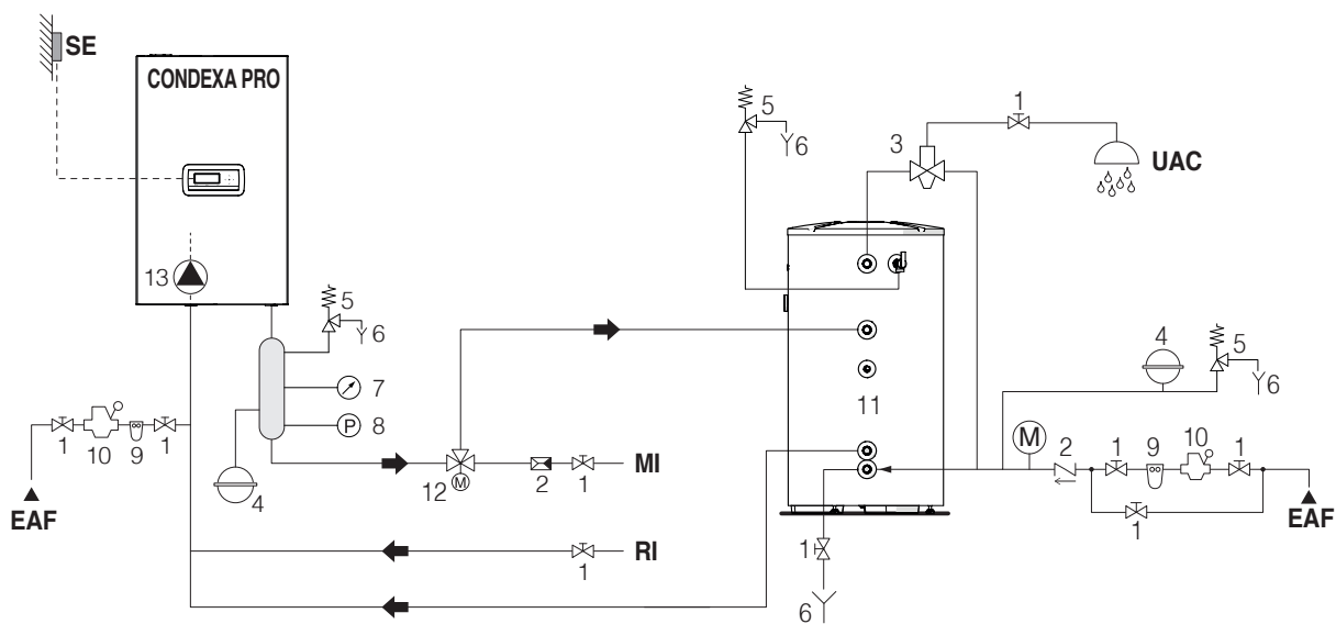
Schema 2: Kreislauf mit direkt an die Heizanlage und BWW-Behälter angeschlossenem Wärmemodul (prüfen, ob die Förderhöhe der Pumpe ausreichend ist, um eine angemessene Zirkulation zu gewährleisten)
