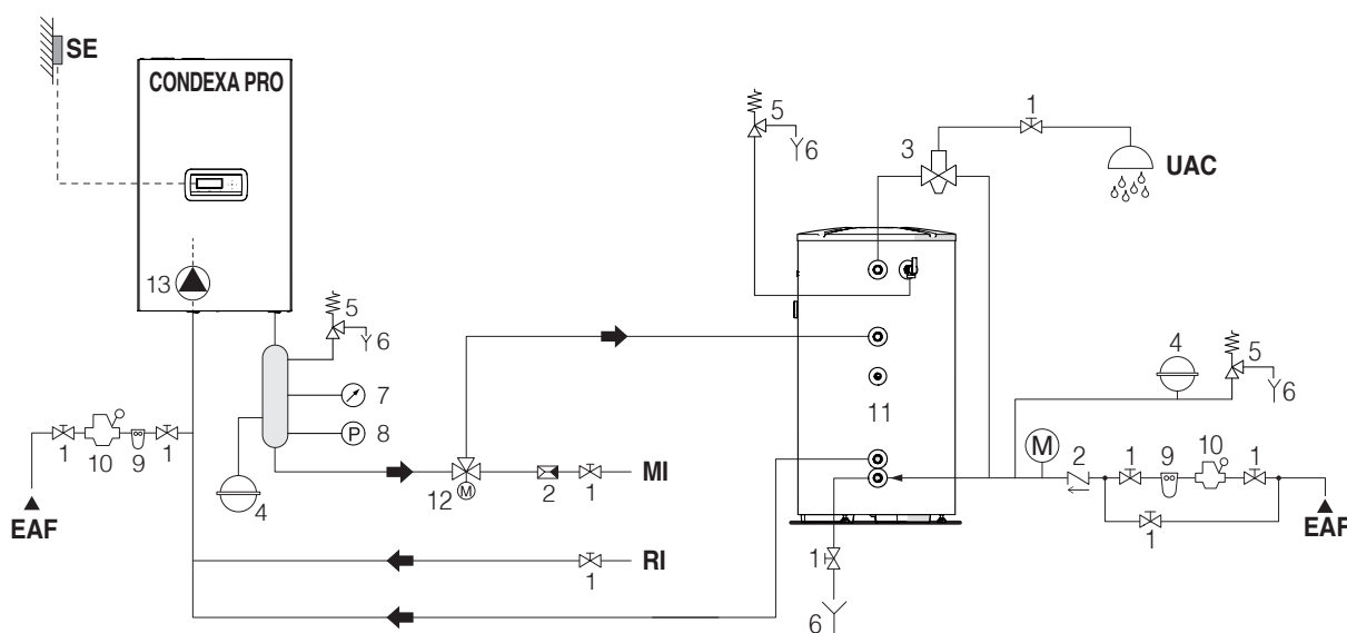
Схема 2: контур теплового модуля, подключенный непосредственно к отопительной системе и бак ГВС (убедитесь, что напор насоса обеспечивает достаточную циркуляцию)
