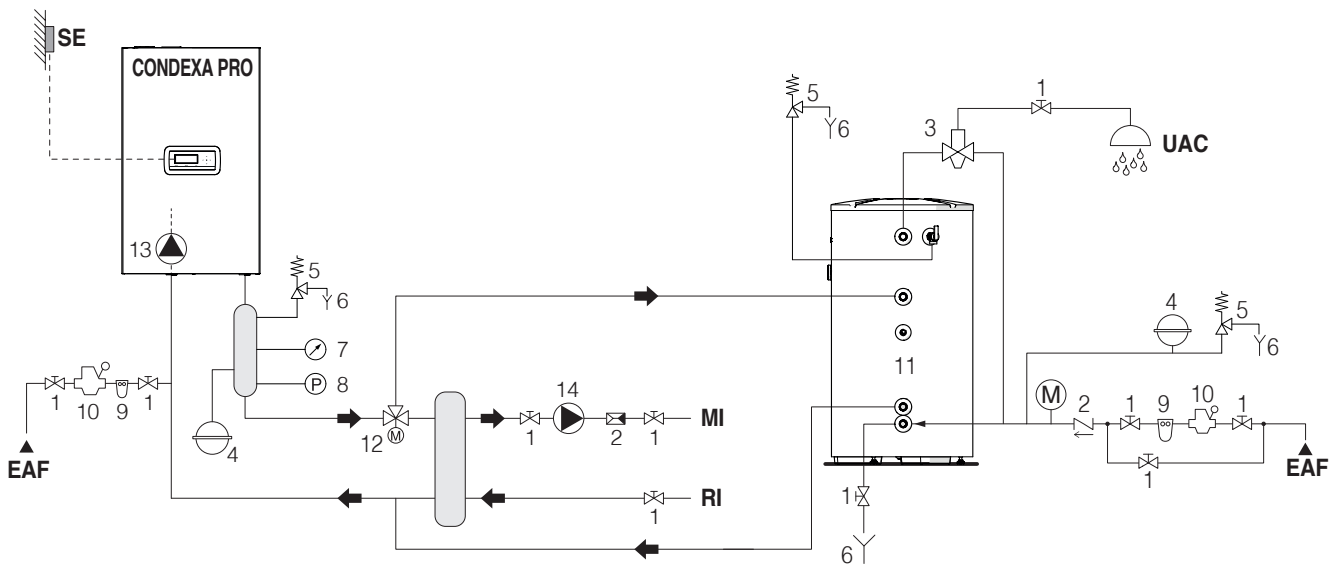
Schema 5: Kreislauf mit Wärmemodul, das mittels Trennstation an der Heizanlage und am BWW-Behälter angeschlossen ist
