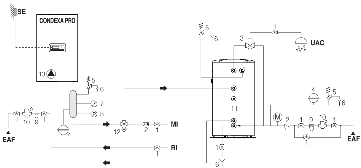
Schema 2: Kreislauf mit direkt an die Heizanlage und BWV-Behälter angeschlossenem Wärmemodul (prüfen, ob die Förderhöhe der Pumpe ausreichend ist, um eine angemessene Zirkulation zu gewährleisten)
