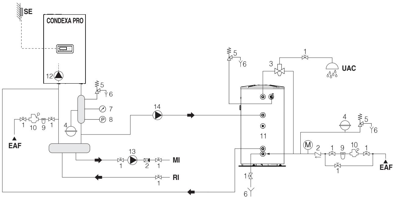
Schema 4: Kreislauf mit Wärmemodul, das am BWW-Behälter und mittels Trennstation an der Heizanlage angeschlossen ist
