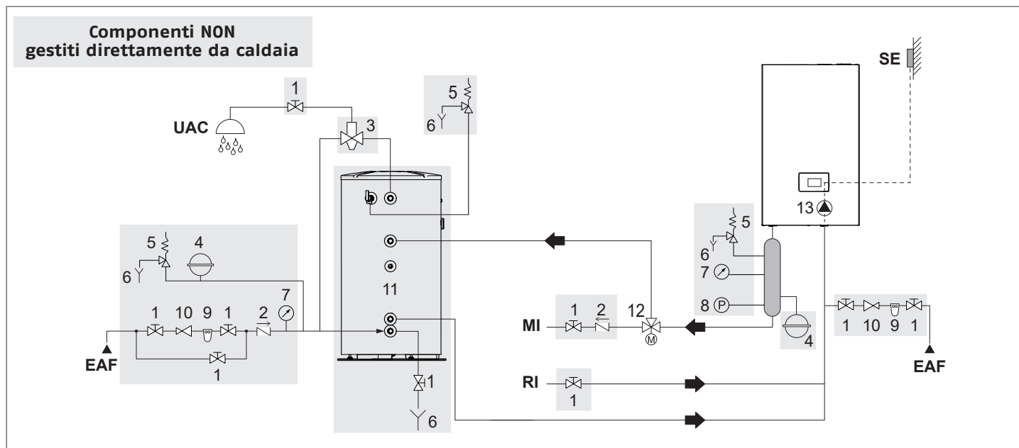
Schema 2: circuito con caldaia collegata direttamente con impianto di riscaldamento e serbatoio A.C.S. (verificare che la prevalenza della pompa sia sufficiente a garantire l'adeguata circolazione)
