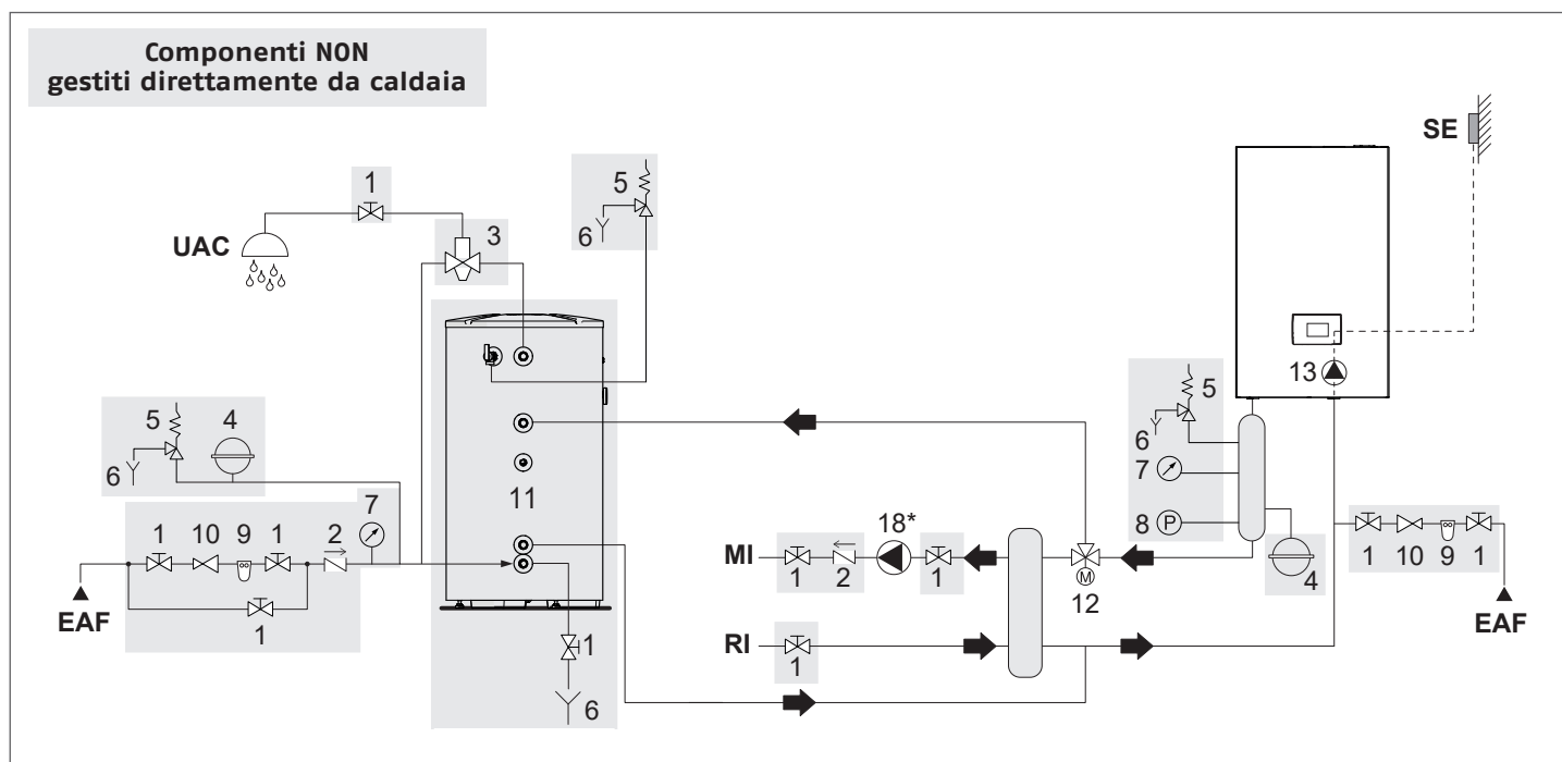
Schema 5: circuito con caldaia collegata con impianto di riscaldamento e serbatoio A.C.S tramite separatore
