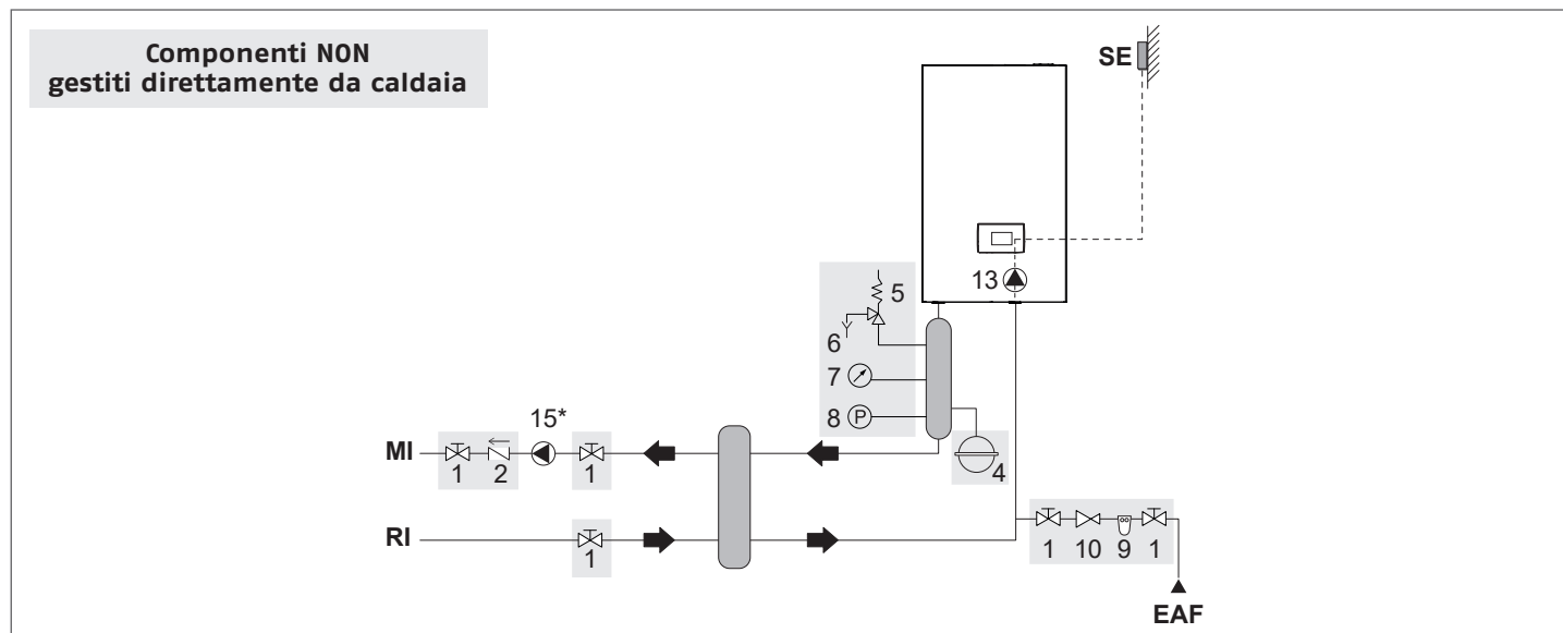
Schema 4: circuito con caldaia collegata con serbatoio A.C.S. e con impianto di riscaldamento tramite separatore
