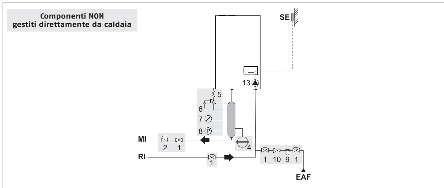
Schema 2: circuito con caldaia collegata direttamente con impianto di riscaldamento e serbatoio A.C.S. (verificare che la prevalenza della pompa sia sufficiente a garantire l'adeguata circolazione)
