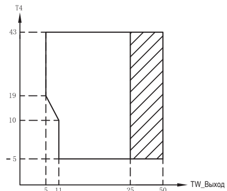
Шaded area: Рабочий диапазон через тепловой насос с возможным ограничением и защитой.
