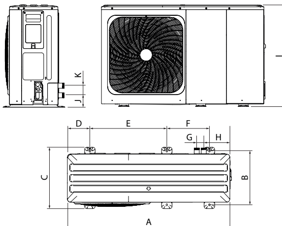
8/10/12/14/16 kW (dimensions en mm)
