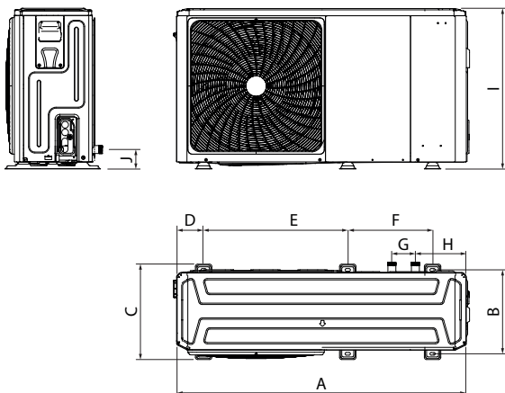
4/6 kW (dimensions en mm)
