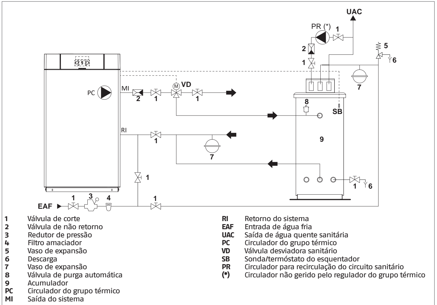
Esquema 2: circuito com grupo térmico ligado diretamente ao sistema de aquecimento e produção de AQS com acumulador e válvula desviadora externa
