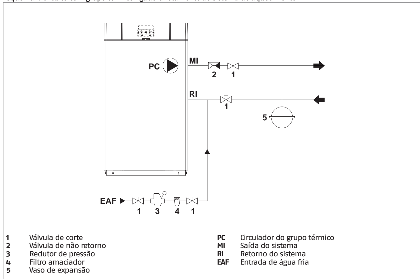
Esquema 1: circuito com grupo térmico ligado diretamente ao sistema de aquecimento
