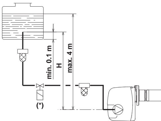
Unter Druck gesetzte Einrohrsysteme
