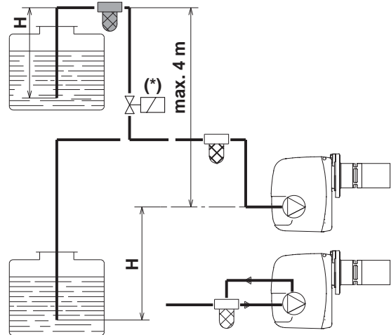
Vakuum-Einrohrsysteme
