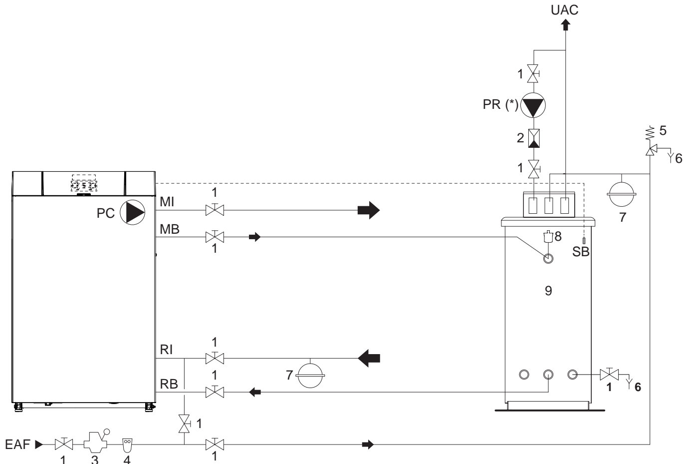
Plan 2: Kreis mit direkt an die Heizungsanlage angeschlossener Wärmeeinheit und Warmwasserbereitung mit Boiler
