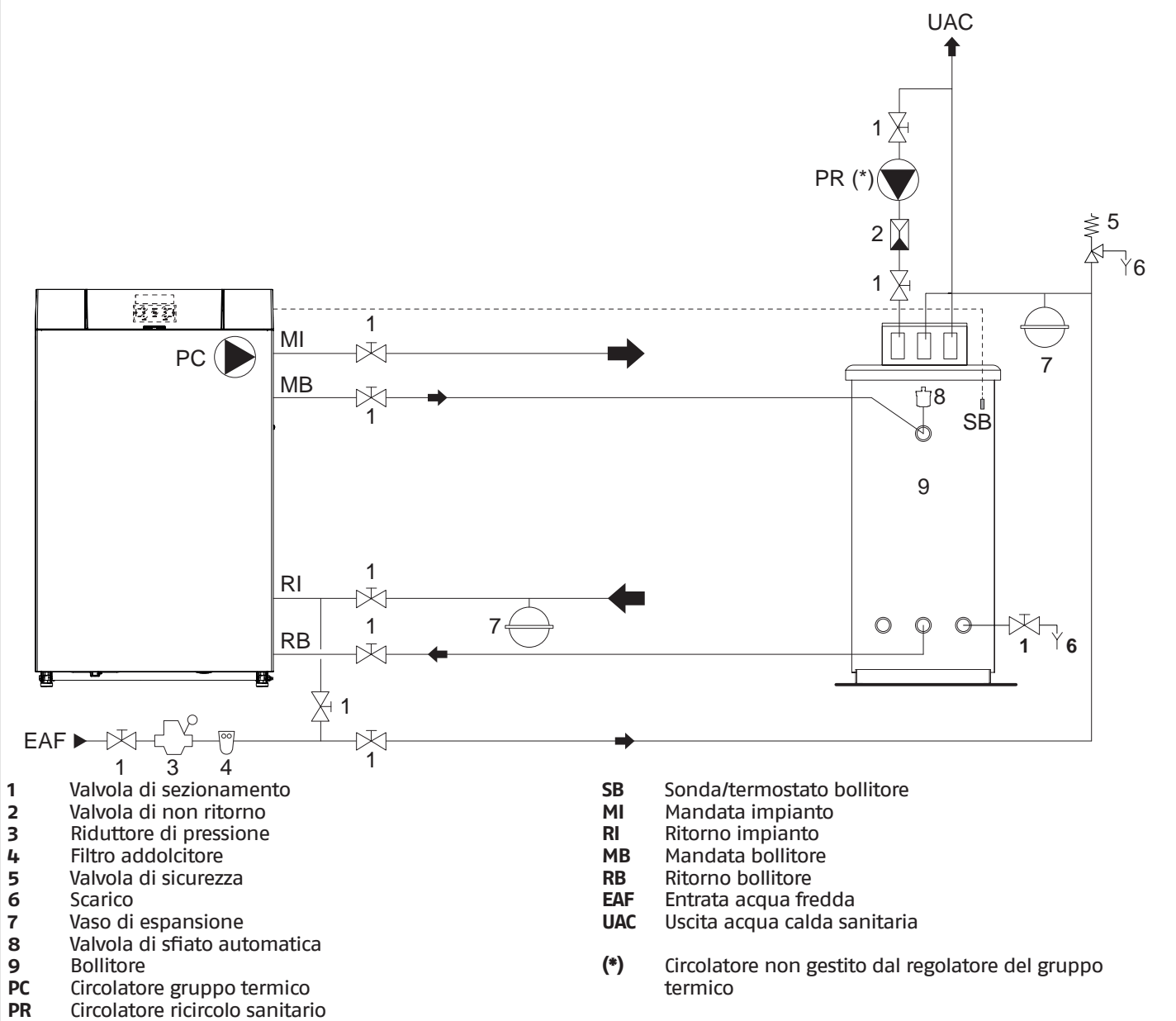
Schema 2: circuito con gruppo termico collegato direttamente all'impianto di riscaldamento e produzione ACS con bollitore
