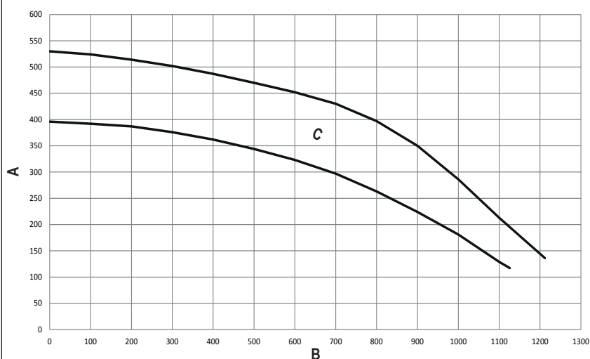
6-metre circulator (factory setted) / pompa de circulație de 6 metri (setare din fabrică) / 6 méteres keringtető szivattyú (gyári beállítás) / Κυκλοφορητής 6 μέτρων (ρυθμιζόμενος από το εργοστάσιο) / Циркуляционная помпа 6 метра (фабрично монтирана) / 6-Meter Umlaufpumpe (Werkseinstellung)
