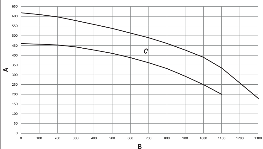
7-metre circulator (accessory) / pompa de circulație de 7 metri (accessoriu) / 7 méteres keringtető szivattyú (tartozék) / Βασικός κυκλοφορητής 7 μέτρων (αξεσουάρ) / Циркуляционная помпа 7 метра (опция) / 7-Meter Umlaufpumpe (Zubehör)
