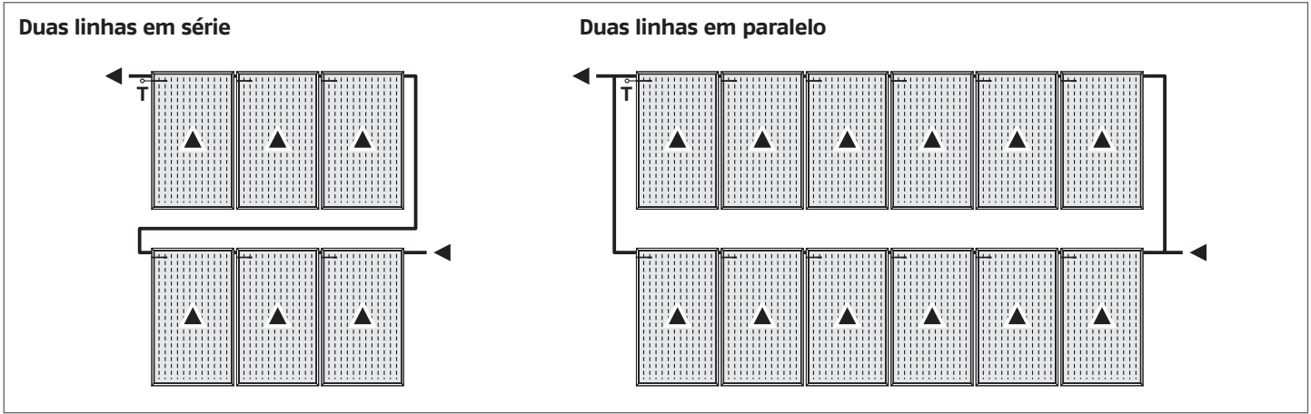
Diâmetro dos tubos de ligação com caudal específico de 30 litros/m²h
