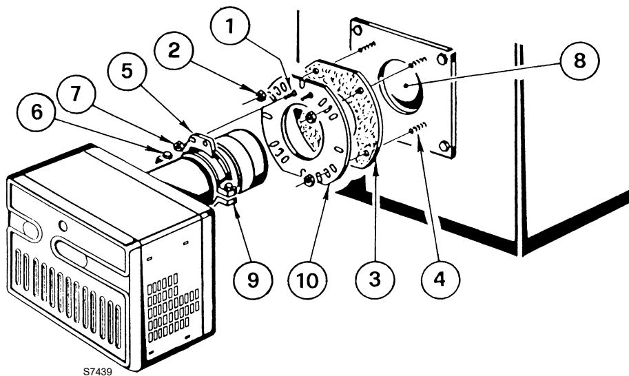
CHAMBRE DE COMBUSTION
