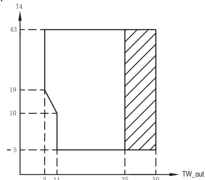
Intervalo de funcionamento por bomba de calor com possível limitação e proteção.
