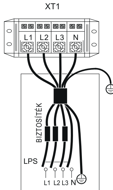
A BELTÉRI EGYSÉG TÁPEGYSÉGE
