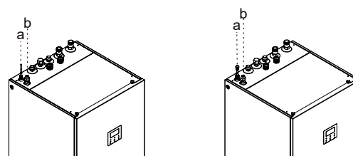
a Conexão de líquido refrigerante b Conexão de gás refrigerante
