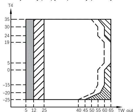
Obszar shaded: Zakres roboczy pompy ciepła z możliwością ograniczenia i zabezpieczenia
