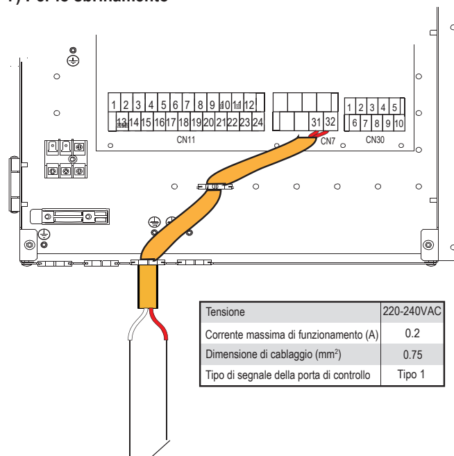
SEGNALE DI RICHIESTA DI SBRINAMENTO
