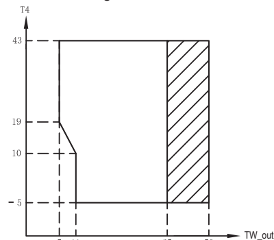
Range di funzionamento mediante pompa di calore con possibile limitazione e protezione.
