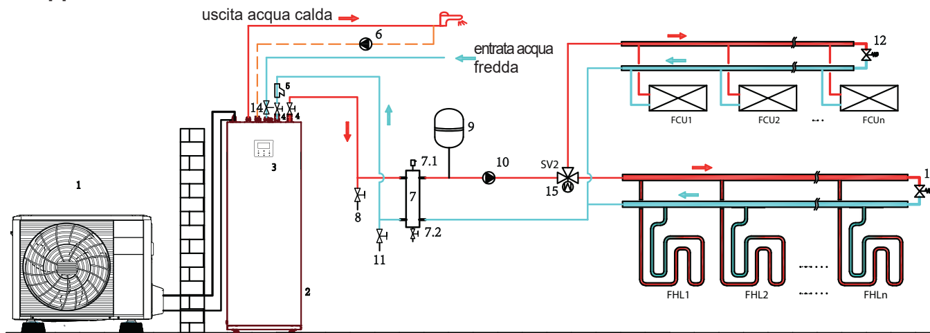
Una zona per impianto a pavimento e ventilconvettori
