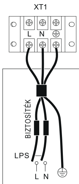
A BELTÉRI EGYSÉG TÁPEGYSÉGE
