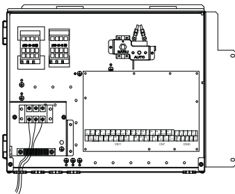
FUENTE DE ENERGÍA DE LA UNIDAD INTERIOR Resistencia eléctrica monofásica de 3 kW estándar
