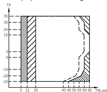
Se l'impostazione IBH/AHS è valida, si accende solo IBH/AHS; Se l'impostazione IBH/AHS non è valida, si accende solo la pompa di calore, potrebbero verificarsi limitazioni e protezioni durante il funzionamento della pompa di calore. La pompa di calore si spegne, si accende solo IBH/AHS Range di funzionamento mediante pompa di calore con possibile limitazione e protezione Linea di temperatura massima dell'acqua in ingresso per il funzionamento della pompa di calore
