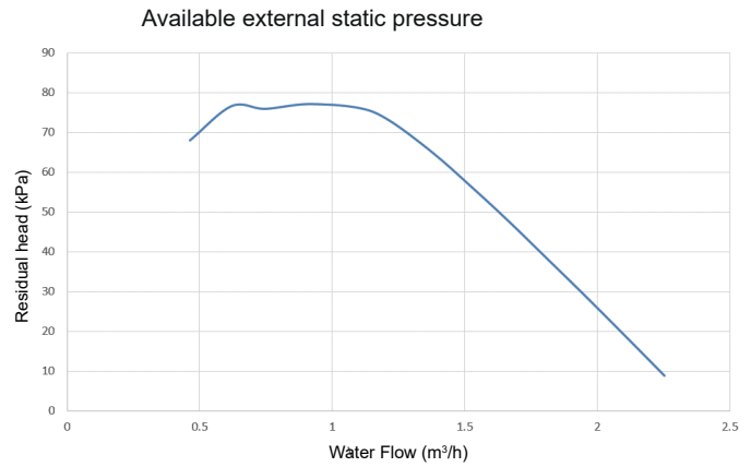
Indoor unit 240L
