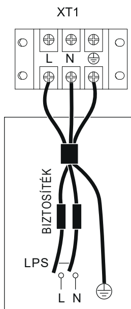
A BELTÉRI EGYSÉG TÁPEGYSÉGE
