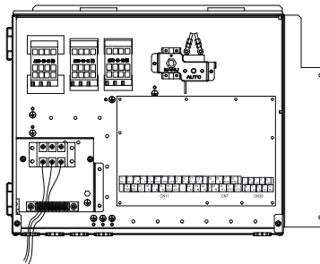
VOEDING BINNENUNIT 1-fase 4kW back-upverwarming optioneel
