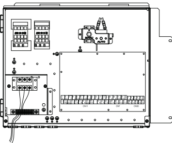
VOEDING BINNENUNIT 1-fase 3kW back-upverwarming standaard
