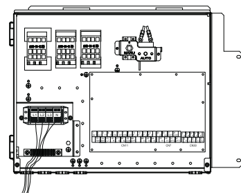
FUENTE DE ENERGÍA DE LA UNIDAD INTERIOR Resistencia eléctrica trifásica de 9 kW estándar
