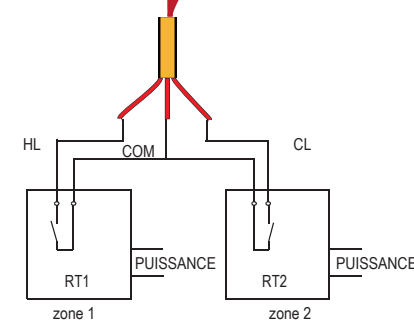
Méthode C (Contrôle double zone)
