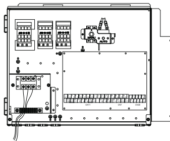
FUENTE DE ENERGÍA DE LA UNIDAD INTERIOR Resistencia eléctrica monofásica de 4kW opcional
