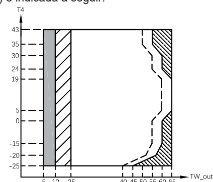
Se a definição IBH/AHS for válida, apenas o IBH/AHS liga. Se a definição IBH/AHS for inválida, apenas a bomba de calor é ligada; casos de limitação e proteção podem ocorrer durante o funcionamento da bomba de calor. Intervalo de funcionamento por bomba de calor com possível limitação e proteção. A bomba de calor desliga-se, apenas o IBH/AHS liga. Linha de temperatura máxima da água de entrada para o funcionamento da bomba de calor.
