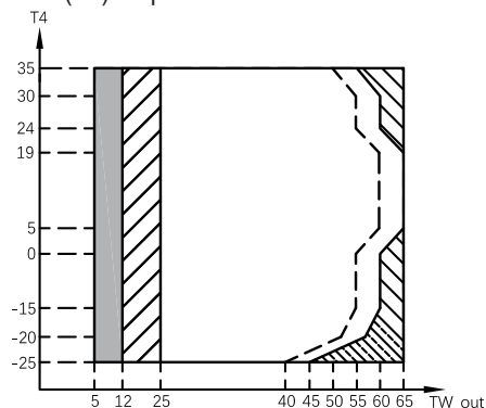
Se a definição IBH/AHS for válida, apenas o IBH/AHS liga. Se a definição IBH/AHS for inválida, apenas a bomba de calor é ligada; casos de limitação e proteção podem ocorrer durante o funcionamento da bomba de calor. Intervalo de funcionamento por bomba de calor com possível limitação e proteção. A bomba de calor desliga-se, apenas o IBH/AHS liga. Linha de temperatura máxima da água de entrada para o funcionamento da bomba de calor.
