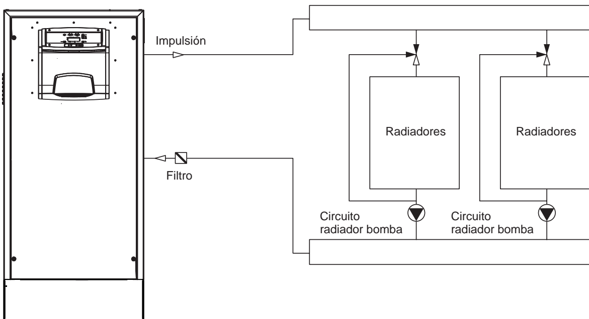
Circuito caldera con un grupo de radiadores. Cada grupo de radiadores tiene su propio mando sensor externo. La curva de la temperatura de impulsión de la caldera es 5 grados superior con respecto a la curva más alta de los grupos
