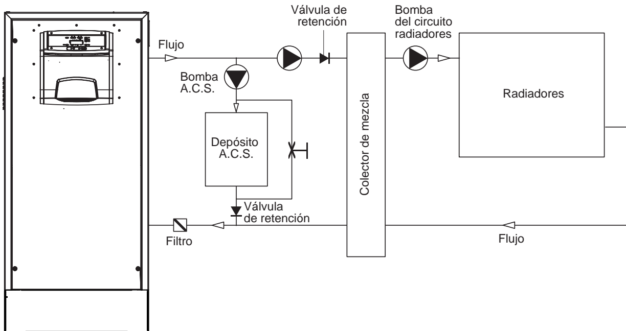
Circuito caldera con bomba A.C.S. (producción caldera > producción A.C.S.) y 1 grupo de radiadores
