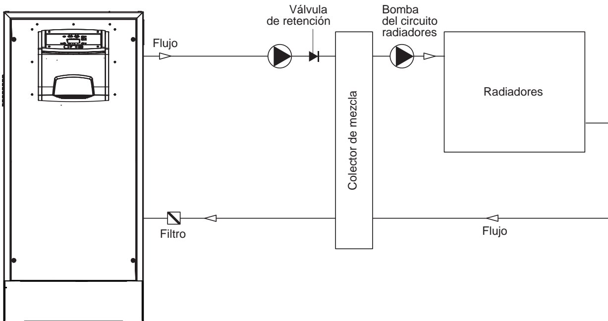
Circuito caldera con un grupo de radiadores Termostato ambiente tipo on/off o de modulación
