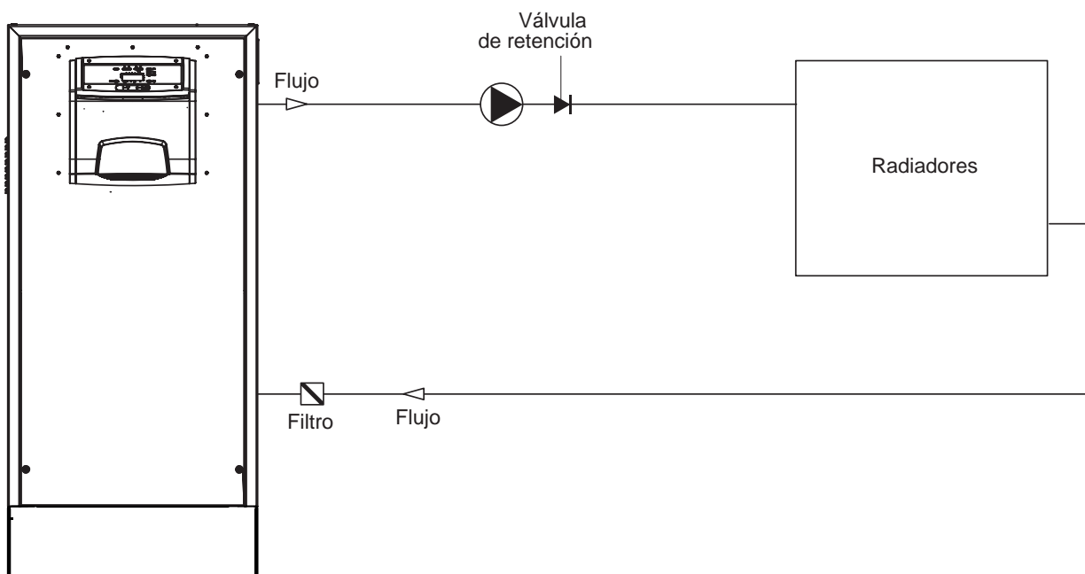
Circuito caldera con un grupo de radiadores
