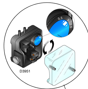
Conexión del manómetro con presostato en absoluto
