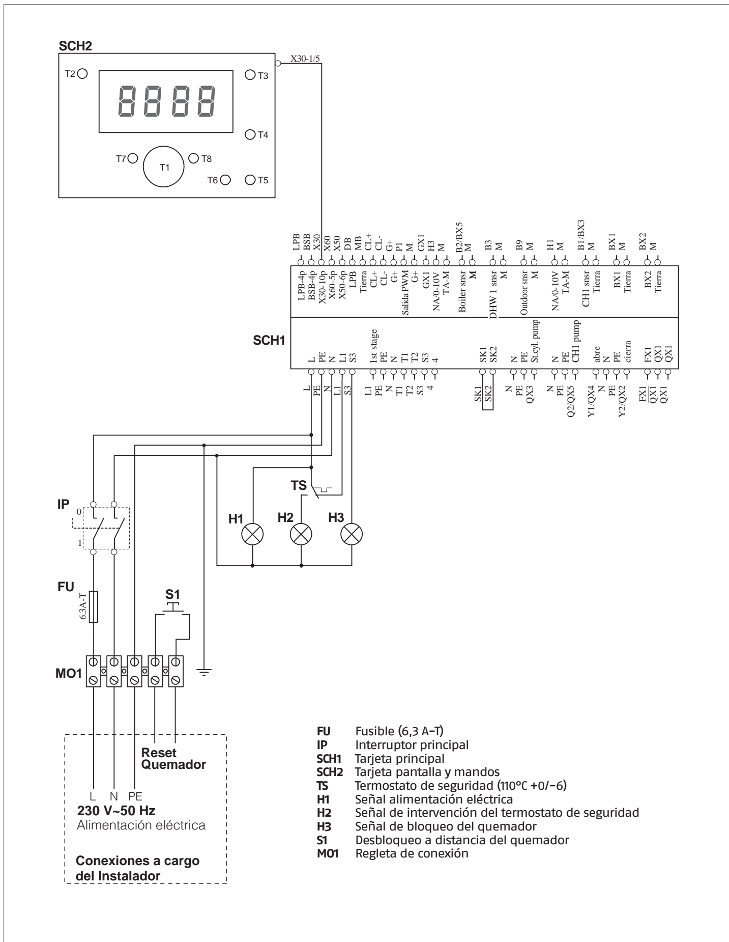
Esquema eléctrico funcional del cuadro eléctrico RIELLOtech CLIMA COMFORT
