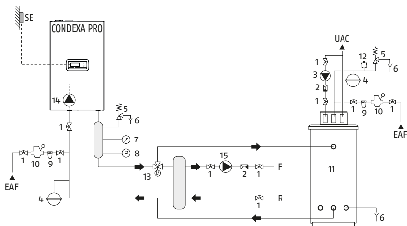
Esquema 5: circuito con módulo térmico conectado al sistema de calefacción y acumulador de ACS mediante separador (la bomba de la caldera garantiza la circulación sólo en el primario).
