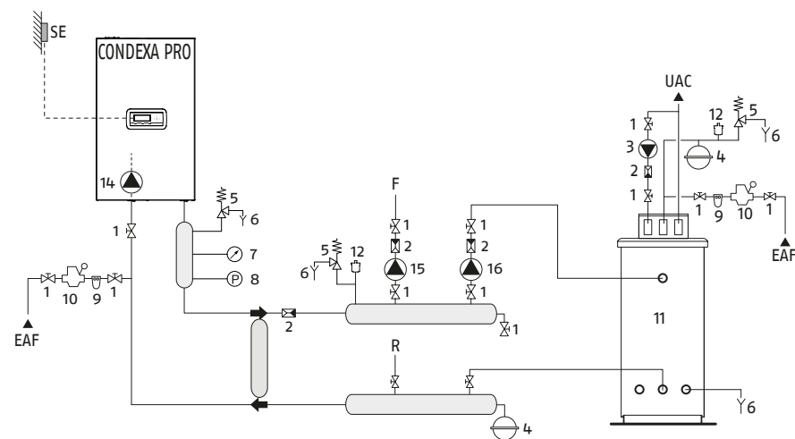
Esquema 6: circuito con módulo térmico conectado al sistema de calefacción y depósito de ACS con colector (en este esquema es posible la simultaneidad). El sistema se construirá únicamente con bombas estándar.
