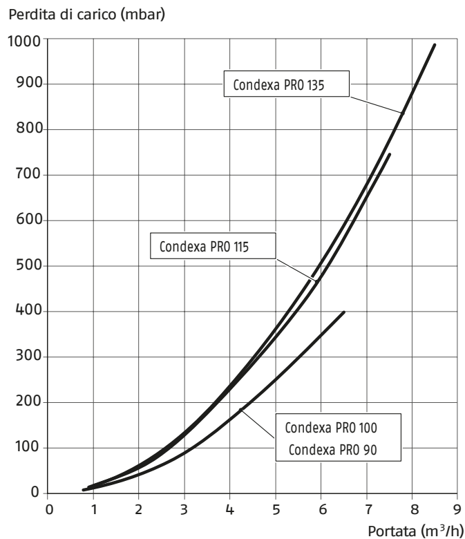
Pérdidas de carga en el lado del agua de los generadores
