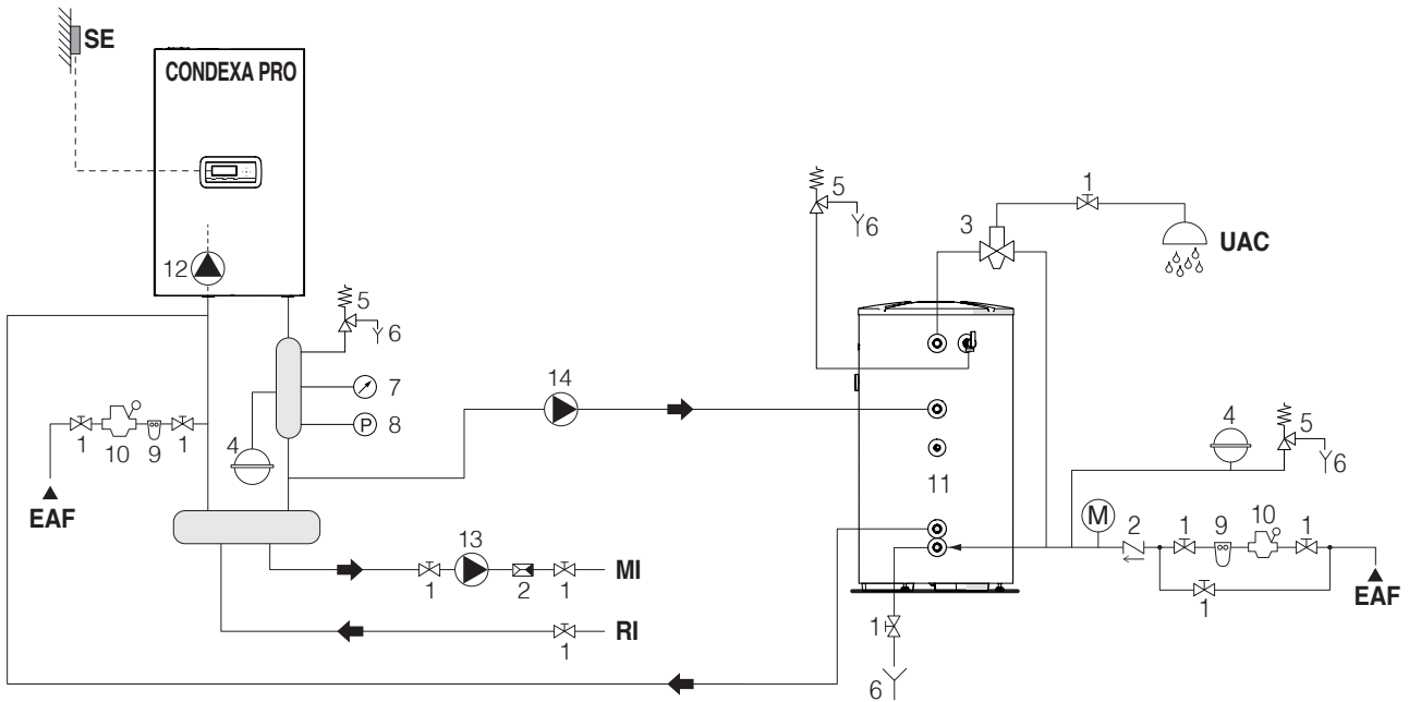
Esquema 4: circuito com módulo térmico ligado ao reservatório de AQS e à instalação de aquecimento através de um separador
